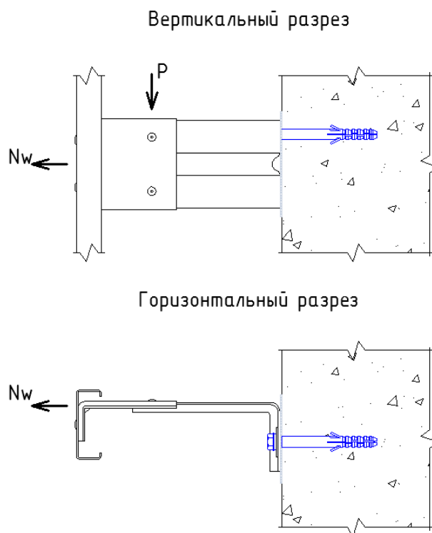
Рисунок 6.3. Конструктивная схема для проверки соединения удлинителя с кронштейном
