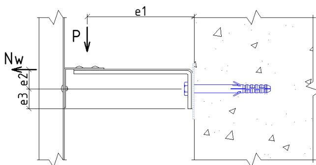
Рисунок 5.2 Расчётная схема проверки анкерного элемента на вырыв
