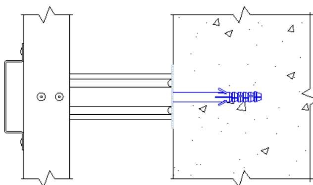
Рисунок 5.3. Конструктивная схема для проверки соединения направляющей с кронштейном
