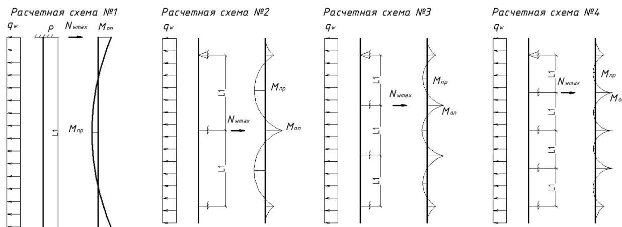
Рисунок 4.9. Расчётные схемы направляющих
