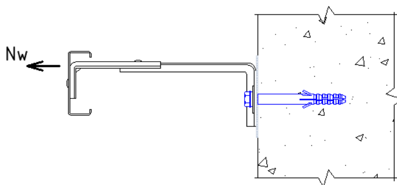
Рисунок 5.6. Конструктивная схема для проверки соединения направляющей с кронштейном
