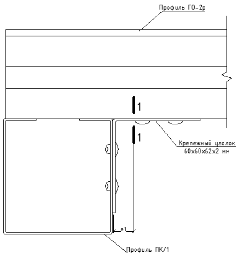
Рис. 7.2. Узел А
